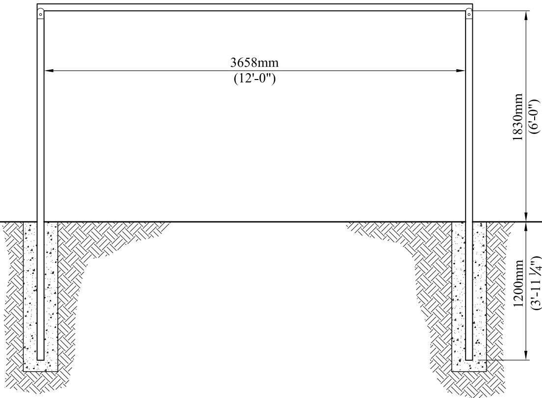
ELEVATION
